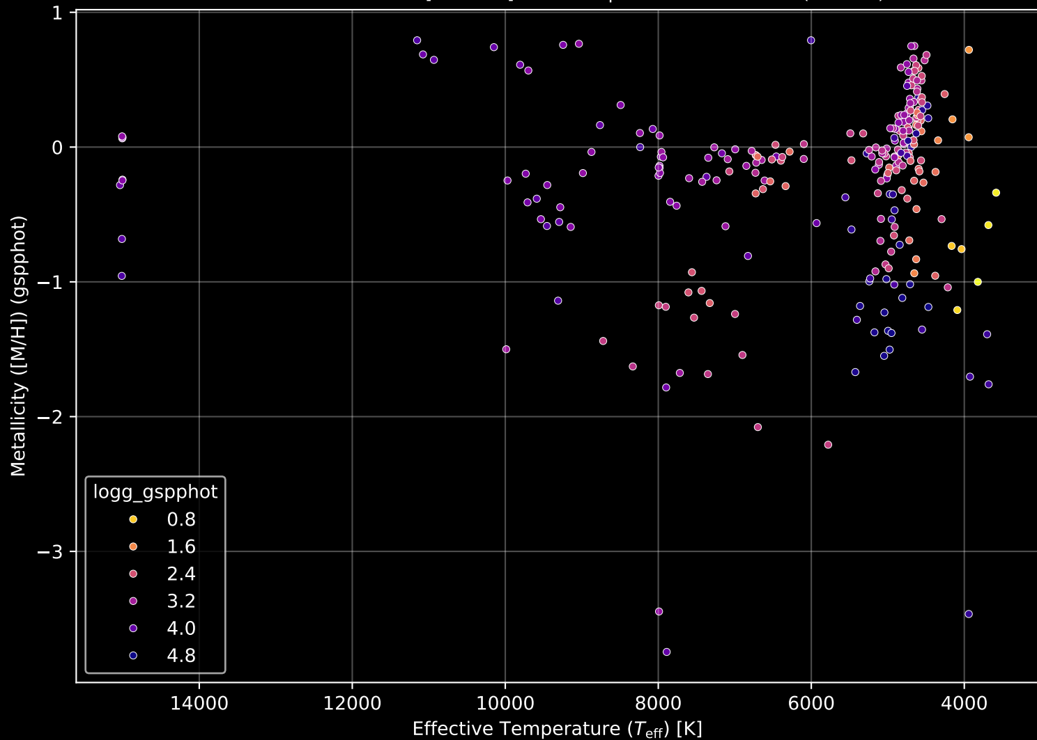
APOGEE DR17 Field: [311+00] Stellar Population Parameters (n= 272)
